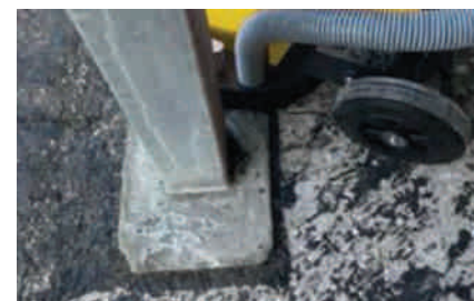
szlifowanie powierzchni blisko krawędzi < 1 cm
